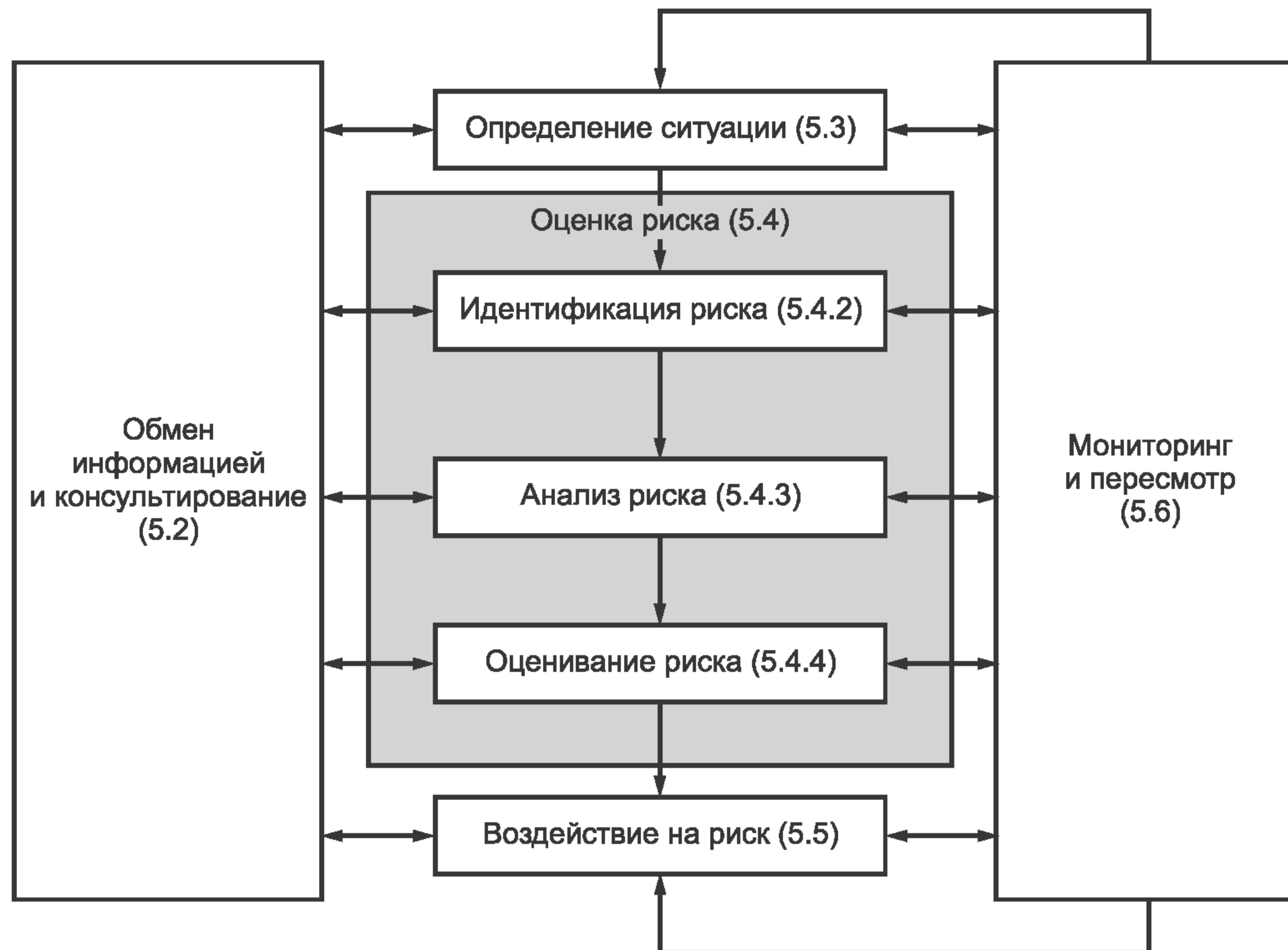
Рисунок 3 — Процесс риск-менеджмента
